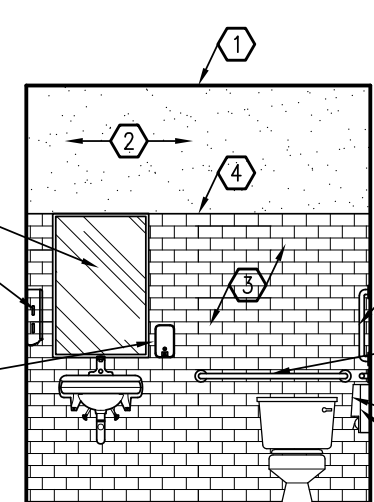
2B TOILET ROOM 109 A-401 1/4"=1'-0"
