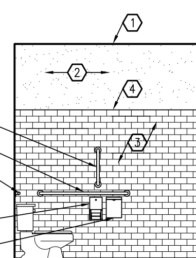
2A TOILET ROOM 109 A-401 1/4"=1'-0"
